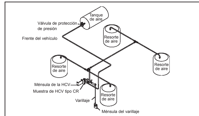
Gráfica 5. Diagrama sencillo de la tubería de una HCV CR
